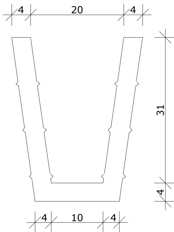
ANSICHT
