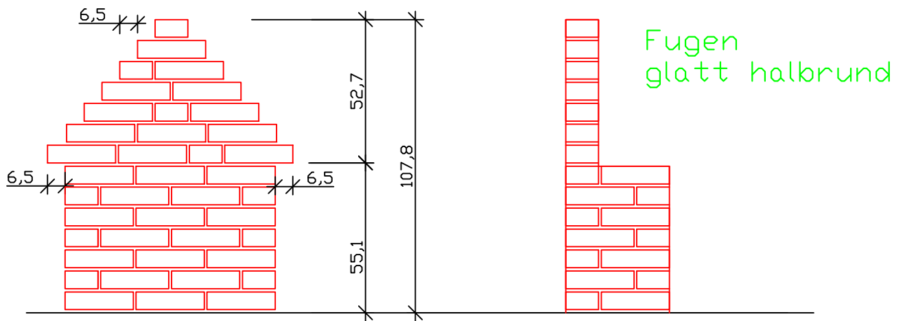
Vorderansicht
