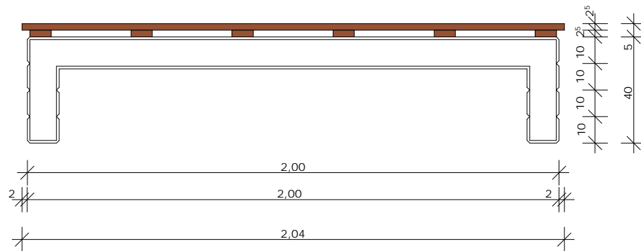
FRONTANSICHT
