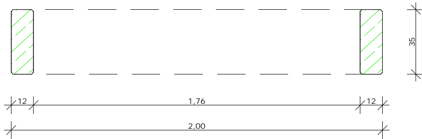
GRUNDRISS
