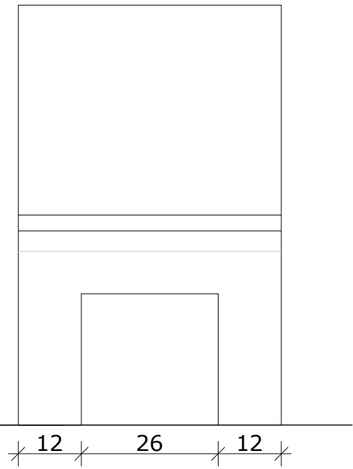
ANSICHT VORDERSEITE
