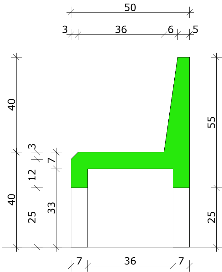
SCHNITT
